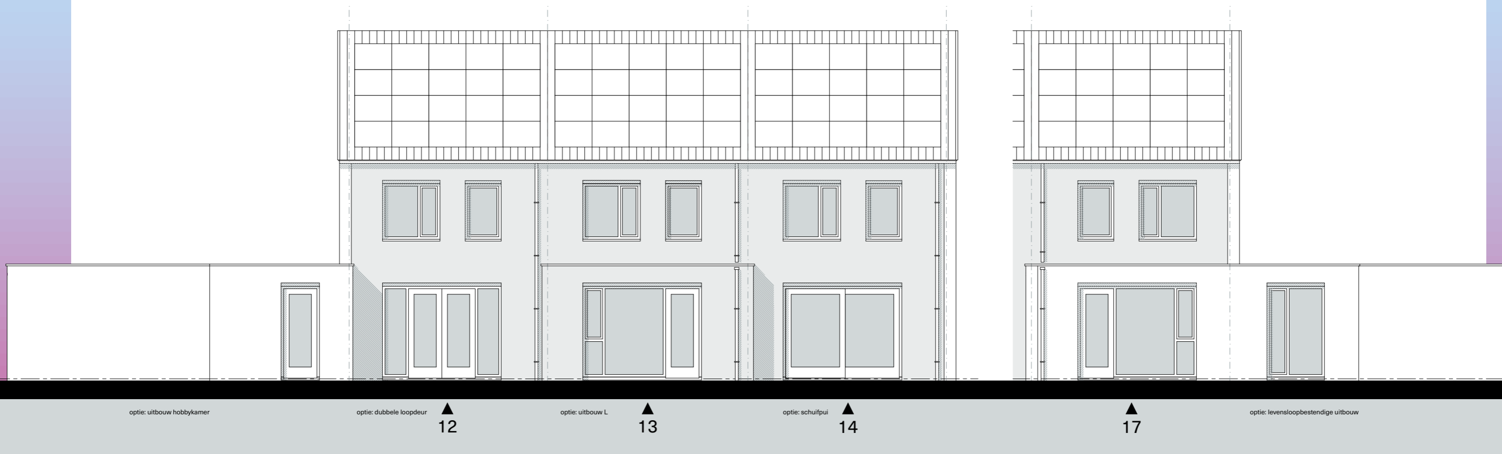
Achtergevel Schaal 1:100
