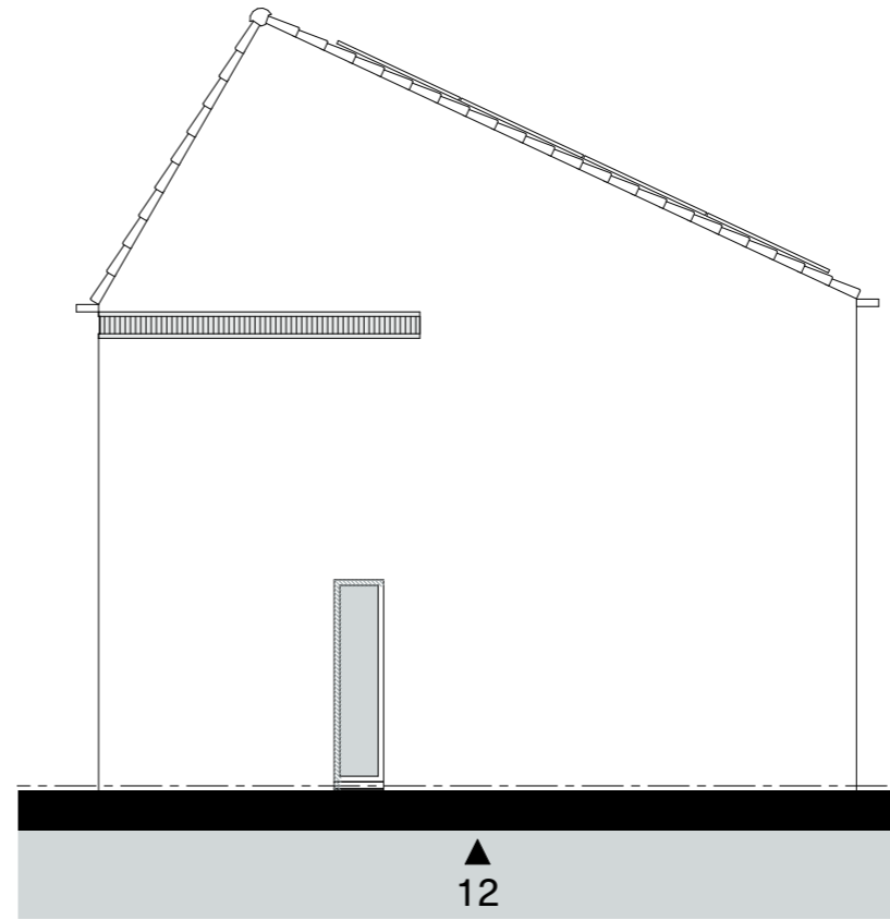
Rechter zijgevel Schaal 1:100
