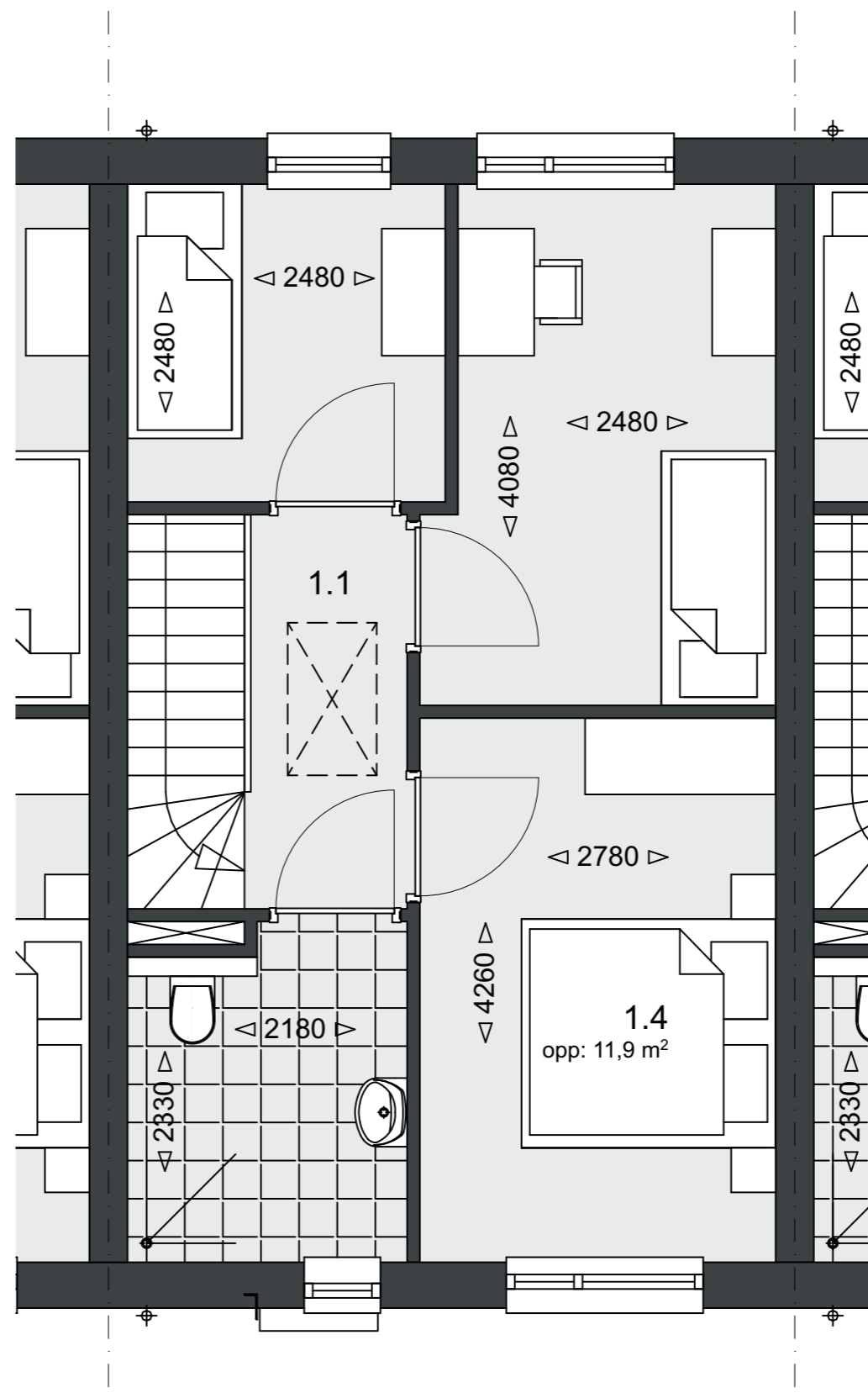
Verdieping 1 Schaal 1:50
