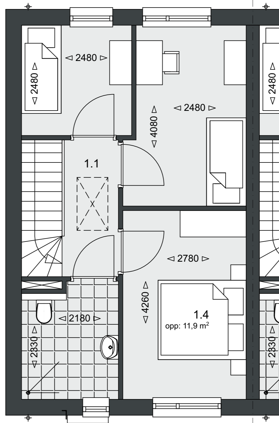
Verdieping 1 Schaal 1:50
