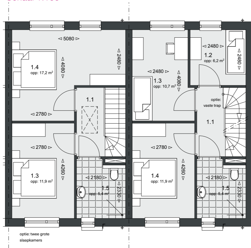
Verdieping 1 Schaal 1:100
