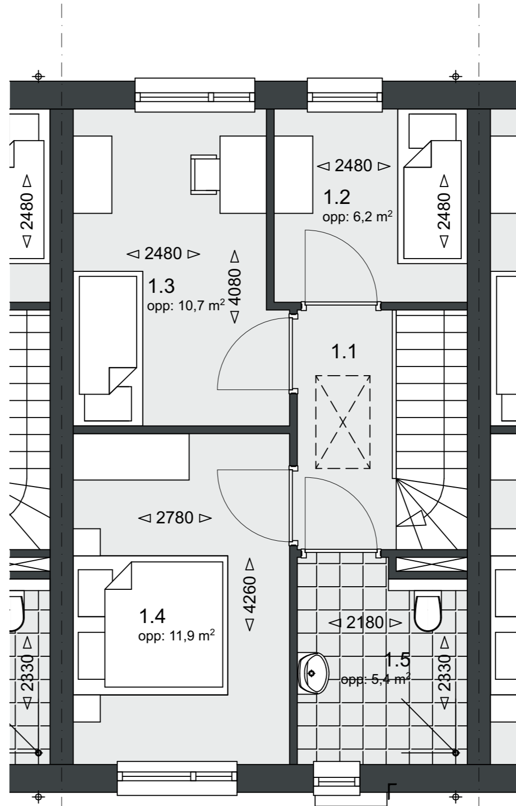
Verdieping 1 Schaal 1:50
