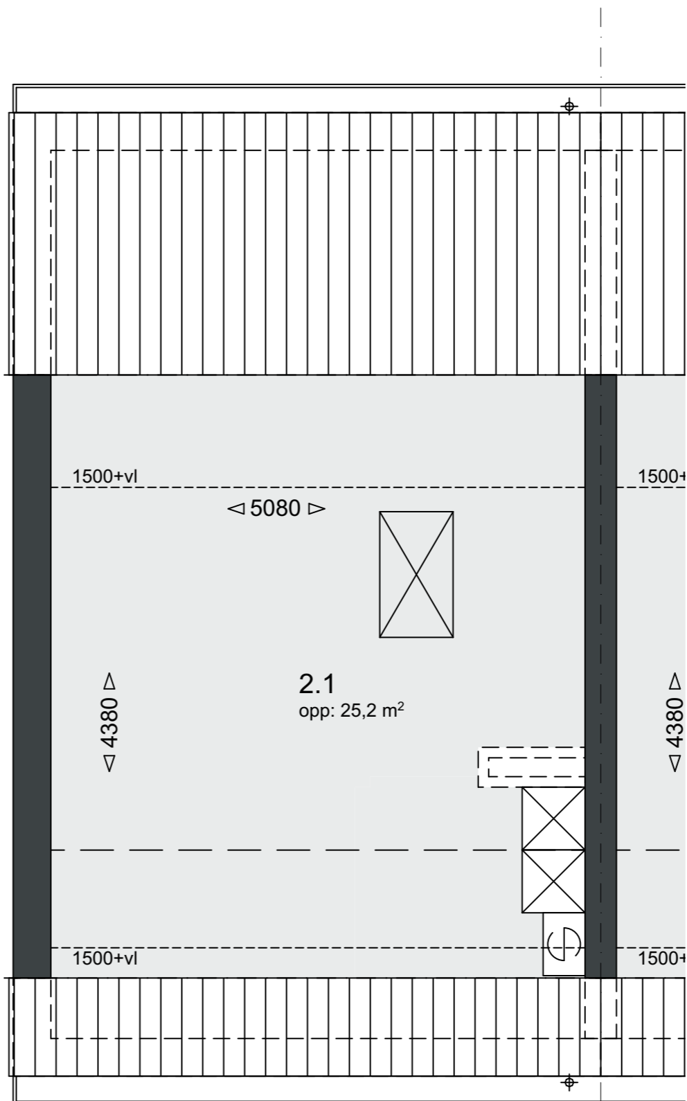
Verdieping 2 Schaal 1:50
