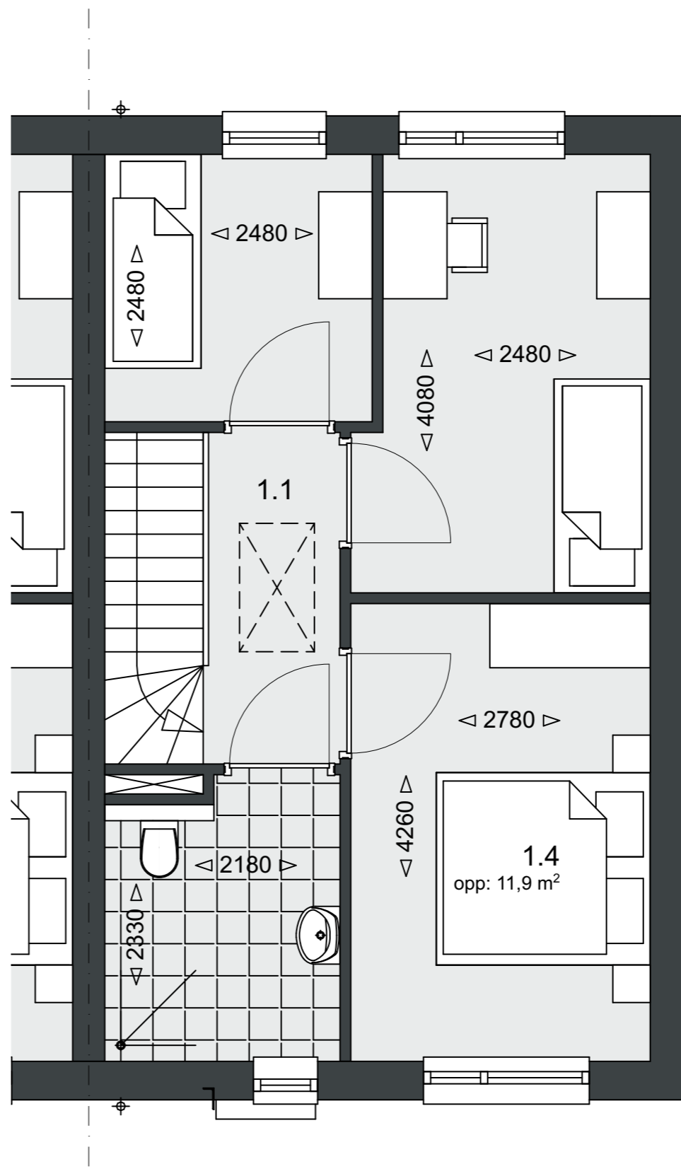
Verdieping 1 Schaal 1:50
