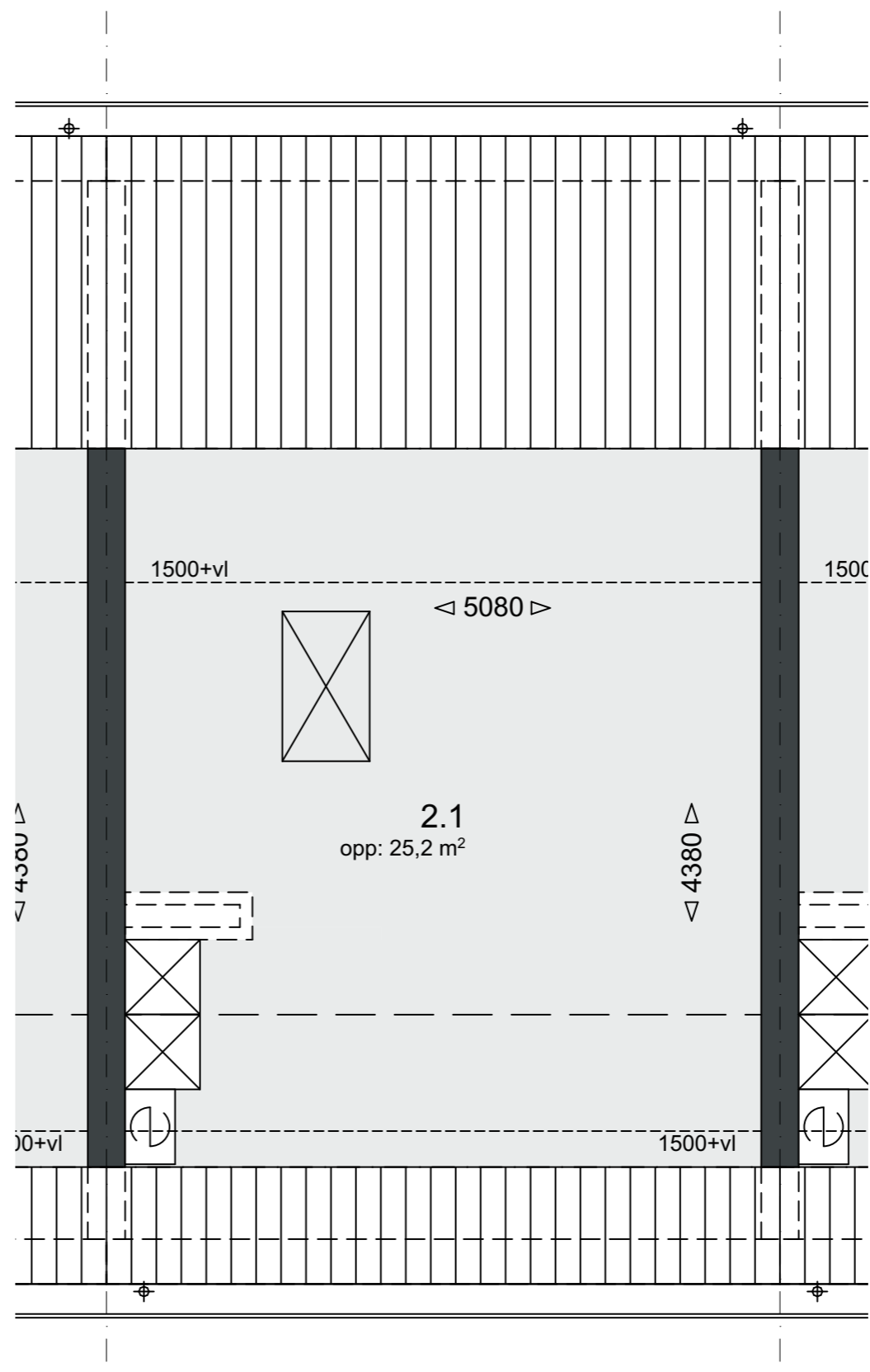
Verdieping 2 Schaal 1:50
