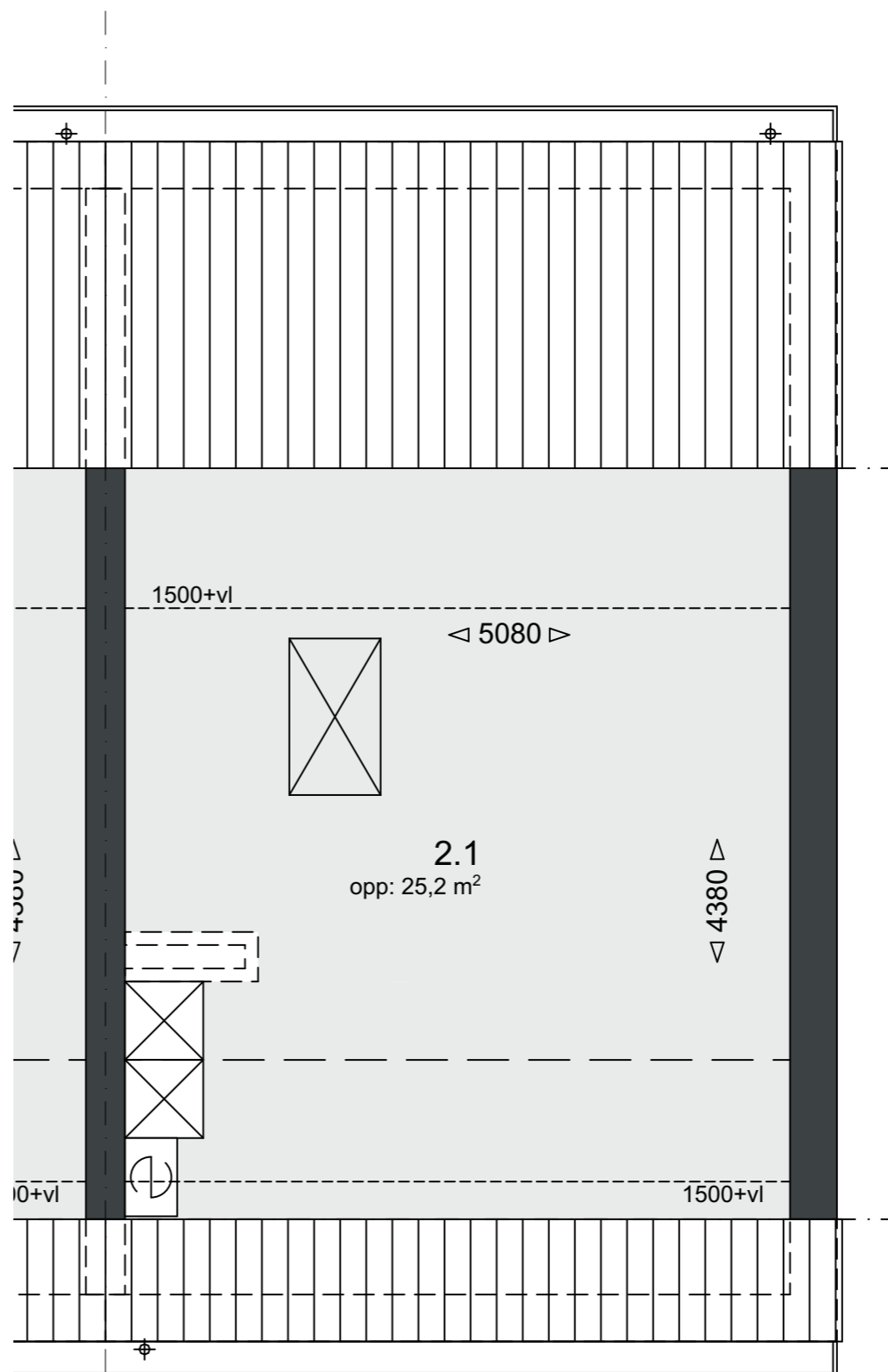
Verdieping 2 Schaal 1:50
