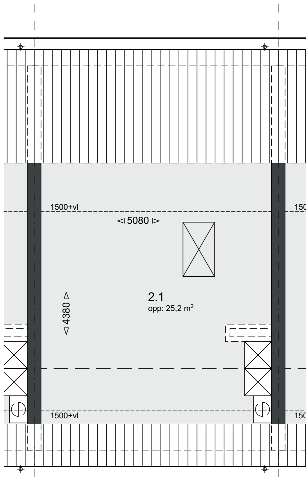
Verdieping 2 Schaal 1:50
