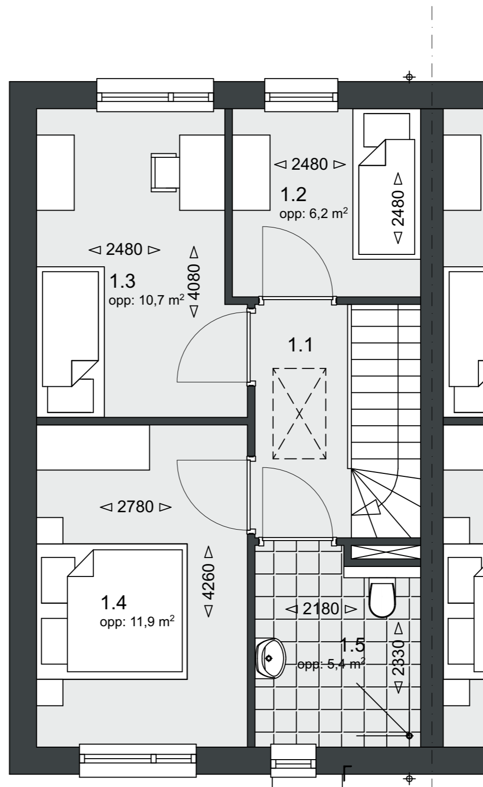
Verdieping 1 Schaal 1:50
