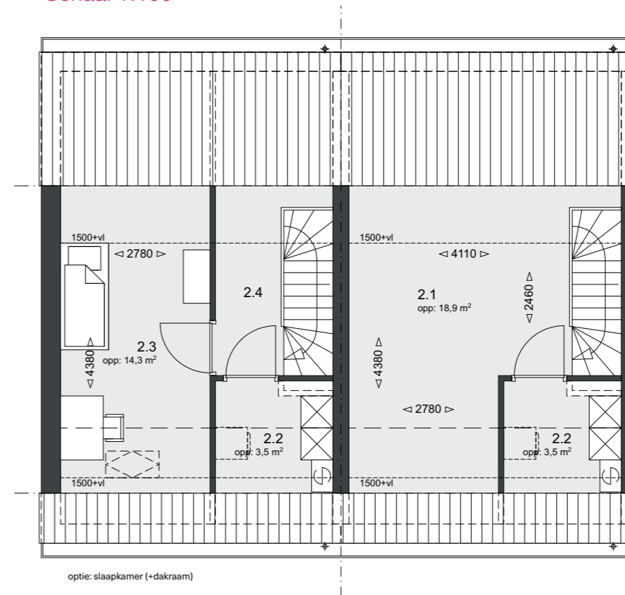
Verdieping 2 Schaal 1:100
