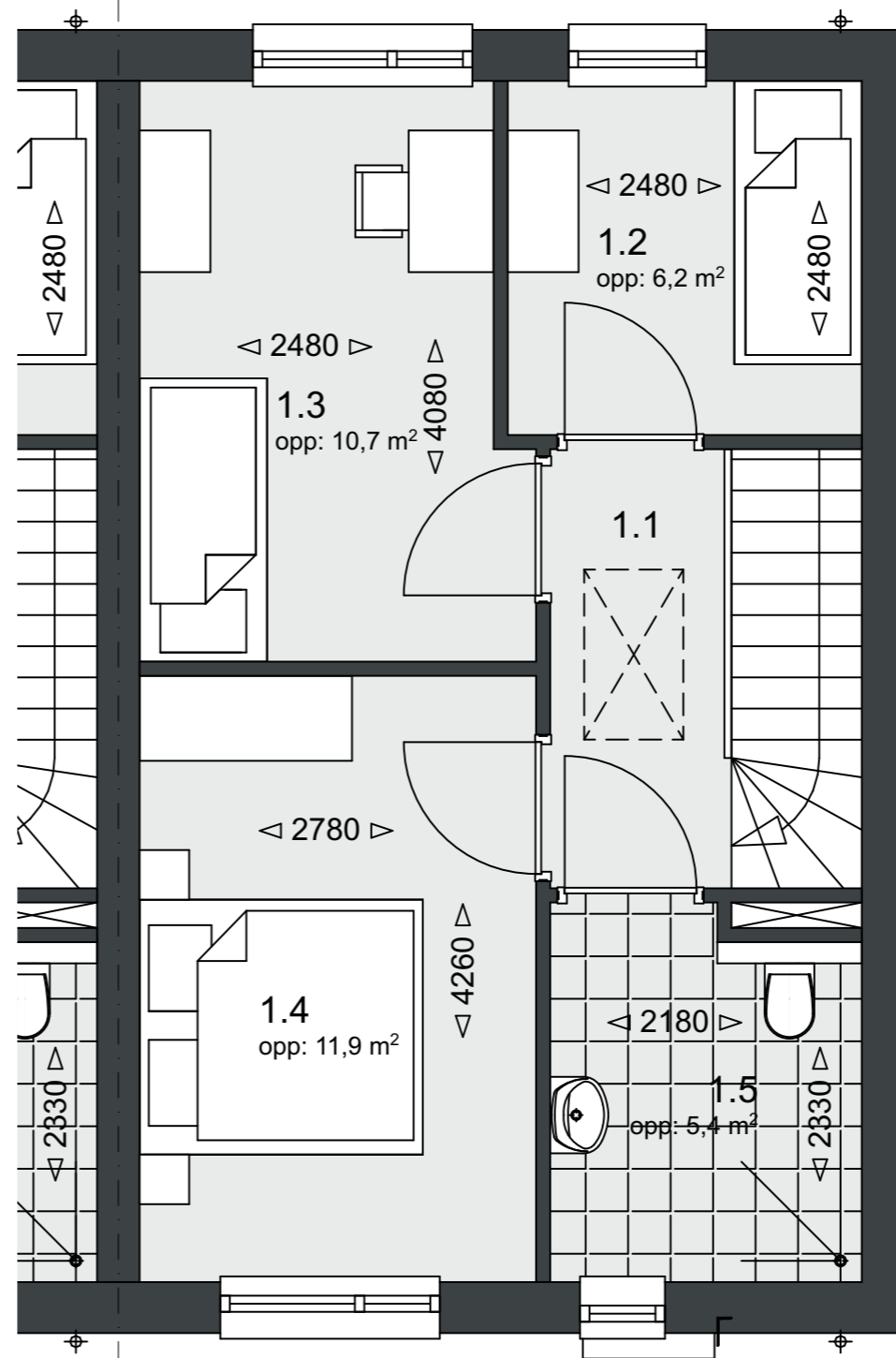
Verdieping 1 Schaal 1:50
